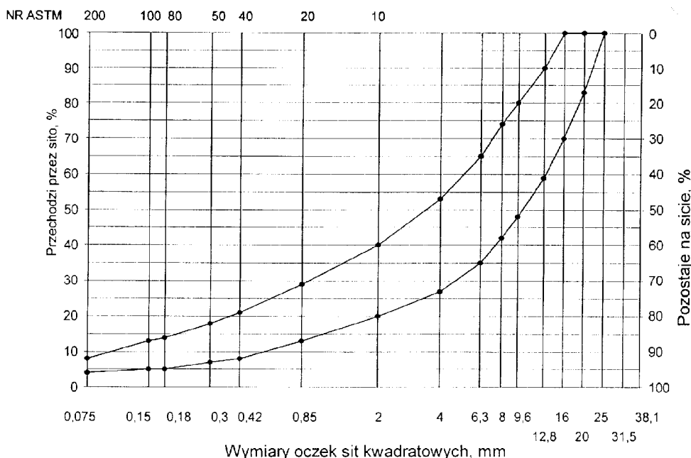
Rys. 1. Krzywe graniczne uziarnienia mieszanki mineralnej BA od 0 do 20 mm podbudowy nawierzchni drogi o obciążeniu ruchem KR 3
