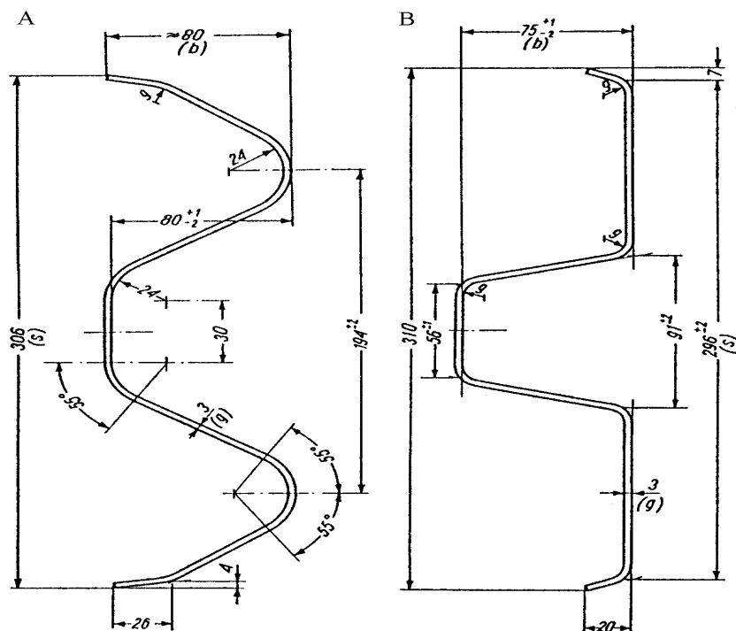
Omówienie różnic taśm stalowych typu A i B
